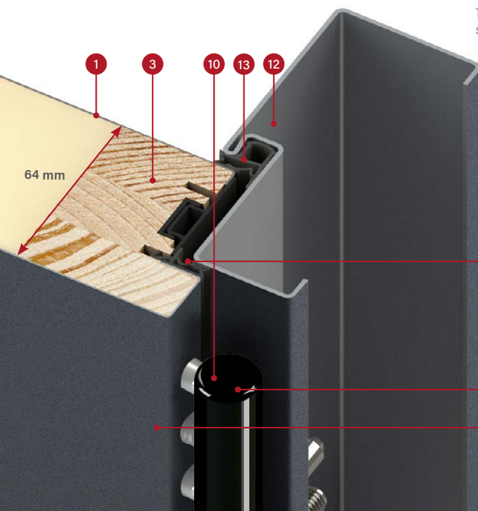
THERMO 64 varčios plieninės staktos skerspjūvis
