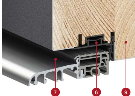
THERMO HOT 78 varčios skerspjūvis su nuleidžiamuoju slenksčiu ir be jo, aliumininis slenkstis
