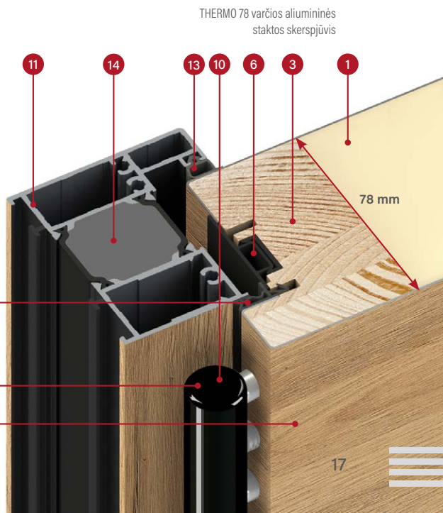
THERMO 78 varčios plieninės staktos skerspjūvis
