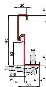
PLIENINĖ KAMPINĖ STAKTA
