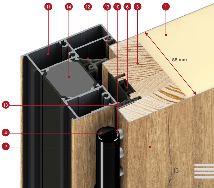
THERMO HOT 88 varčios aliumininės staktos skerspjūvis
