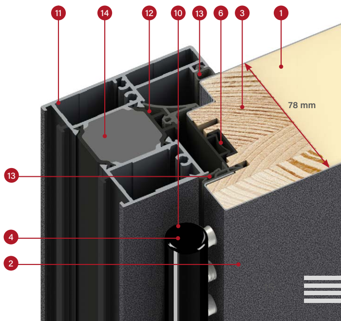
THERMO HOT 78 varčios aliuminės staktos skerspjūvis
