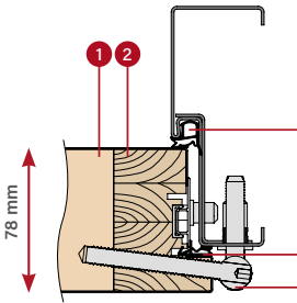
PLIENINĖ STAKTA
