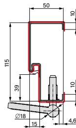
PLIENINĖ STAKTA
